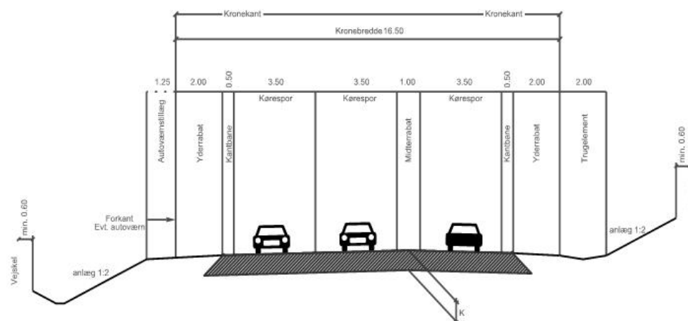
Figur 4.3 Normaltværprofil for 2+1 vej.
