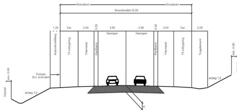
Figur 4.2 Normaltværprofil for 2-sporet vej.
