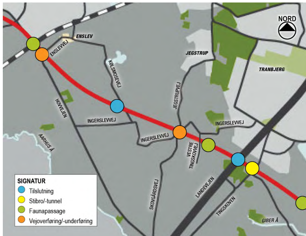
Figur 4.10 Alternativ A mellem Landevejen og Enslevvej.
