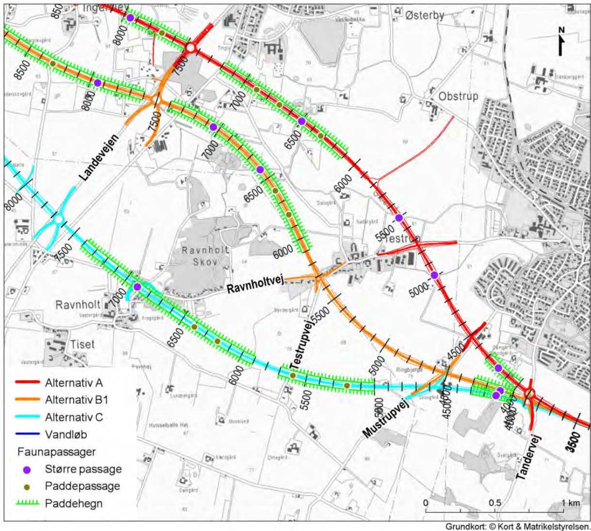
Figur 8.8 Faunapassager indarbejdet i projektet på strækning 2 fra Tandervej til Landevejen. Passagerne er beskrevet under afværgeforanstaltninger for hvert af alternativerne.
